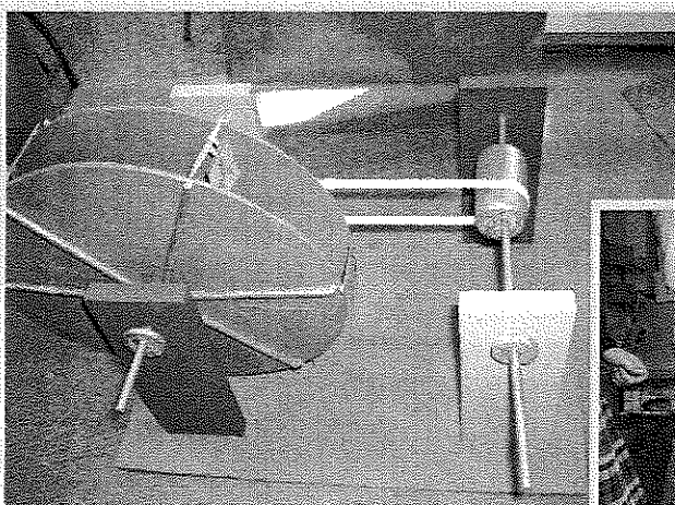
noria con poleas
